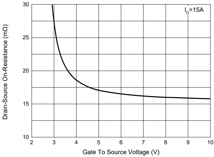
Fig. 3 - R_{DS(ON)} — V_{GS}
