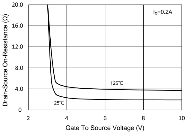
Fig.3 - R_{DS(ON)} - V_{GS}
