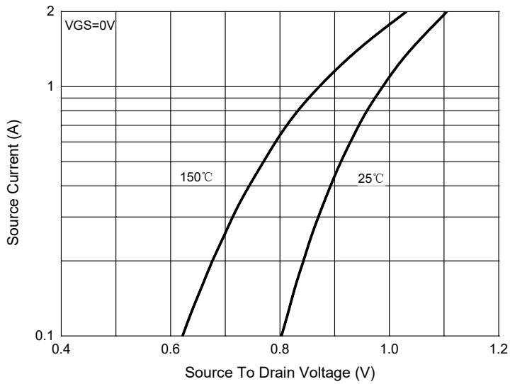
Fig.9 - I_S - V_{SD}
