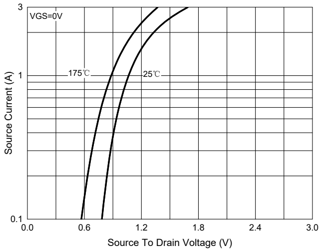
Fig.9 - I_S - V_{SD}
